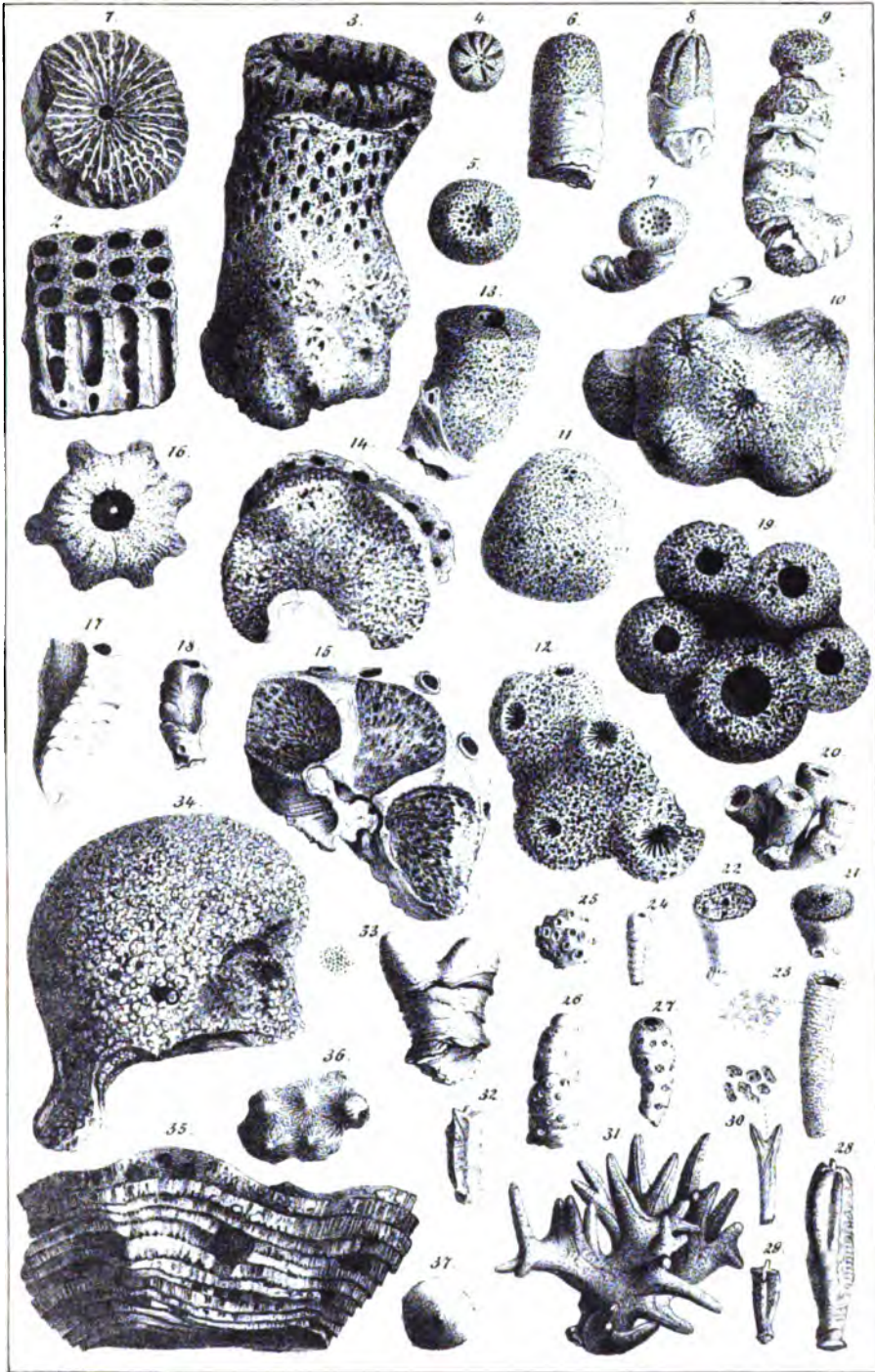
Guonstedt, Jura.
